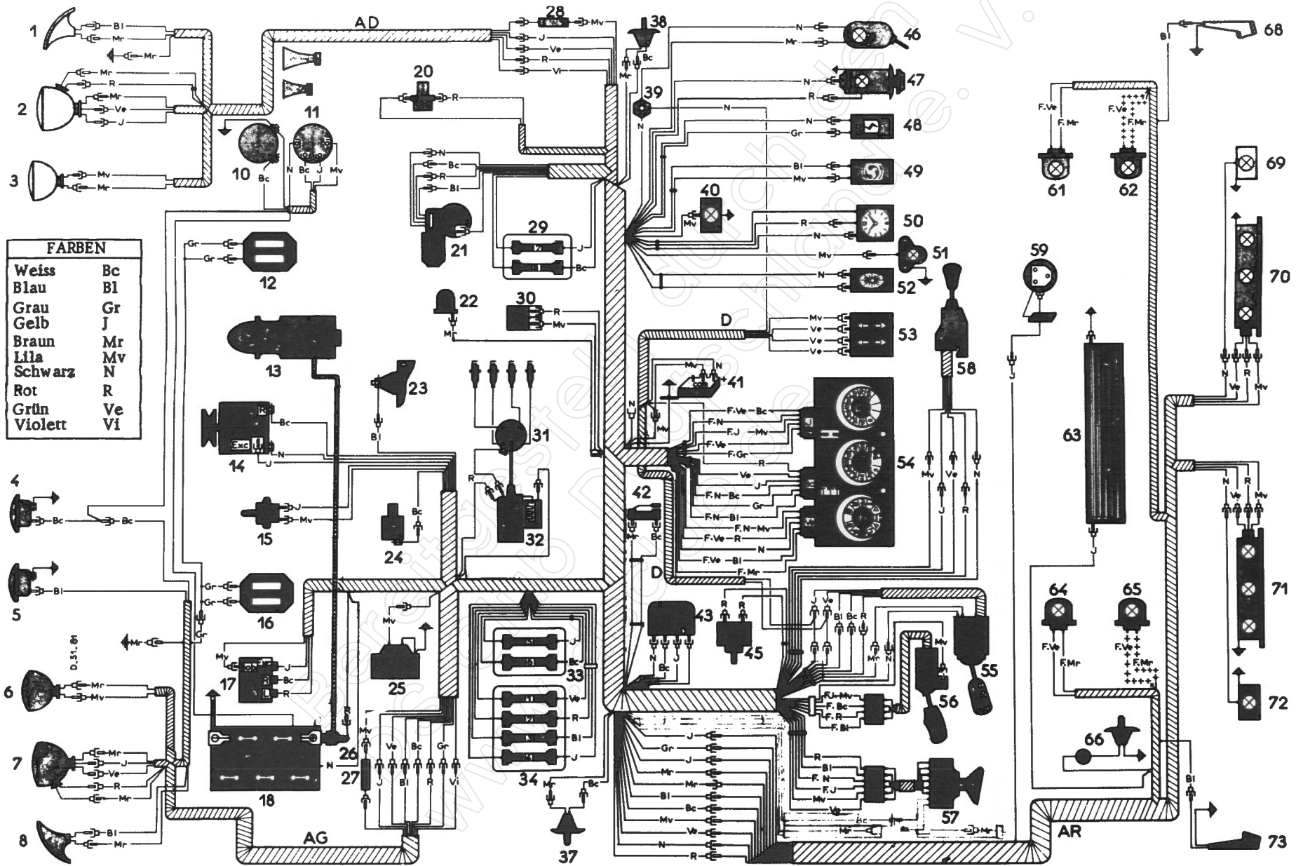
EINBAUSCHEMA
